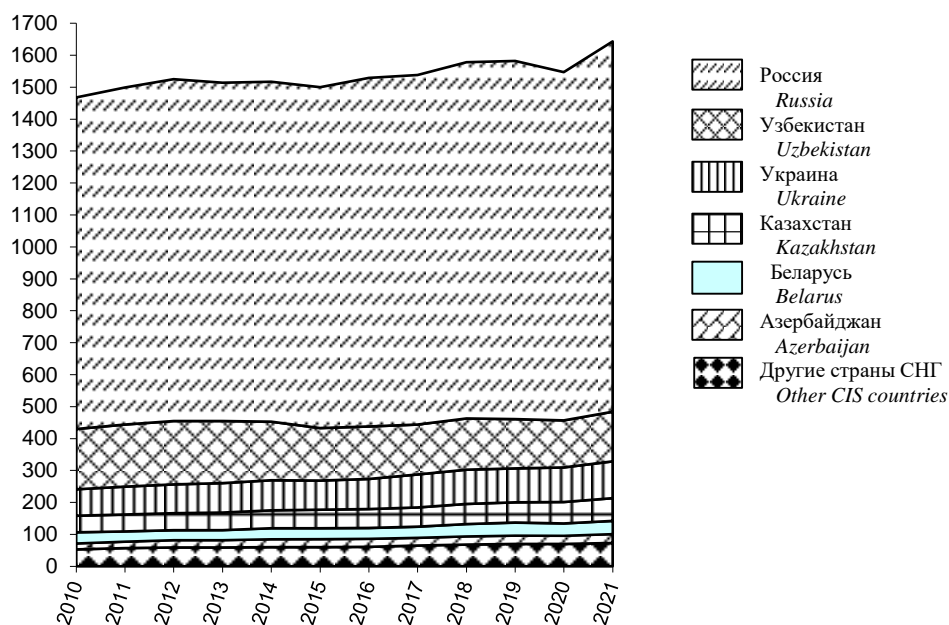
2.2.28. ПРОИЗВОДСТВО ЭЛЕКТРОЭНЕРГИИ (млрд. кВт. ч) 2.2.28. PRODUCTION OF ELECTRIC ENERGY (billion kWh)
