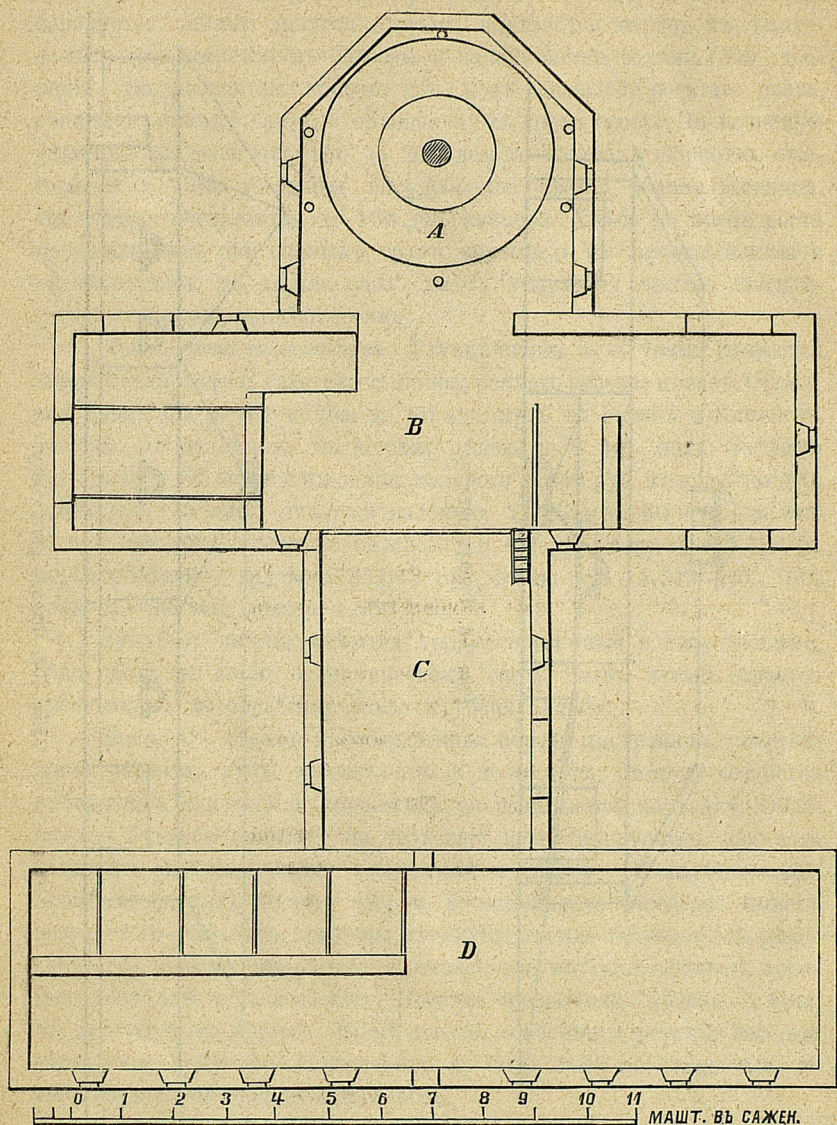
Рис. 1-й. Разрѣзъ риги: A —конный приводъ; B —молотильный сарай; C —отдѣленіе для сортировки зерна; D —амбаръ.
