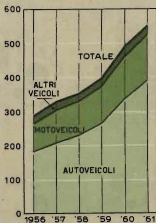
VEICOLI COINVOLTI
