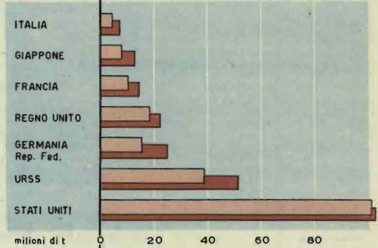
CEMENTO
