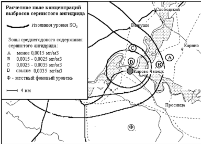
Рис.1. Расчётное поле рассеивания сернистого ангидрида от источников в г.г. Кирове и Кирово-Чепецке.
