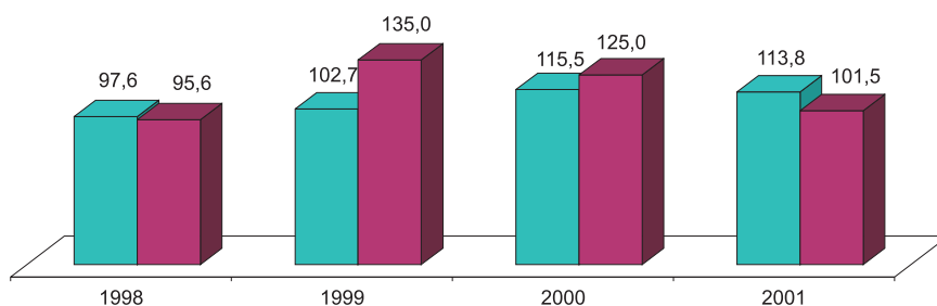
Қазақстан Республикасында табиғи (жанатын) газ өндірудің негізгі көрсеткіштер серпіні Динамика основных показателей добычи природного (горючего) газа Республики Казахстан
