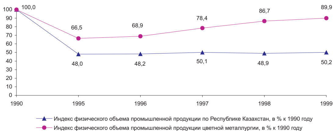
Динамика основных показателей по цветной металлургии и Республике Казахстан
