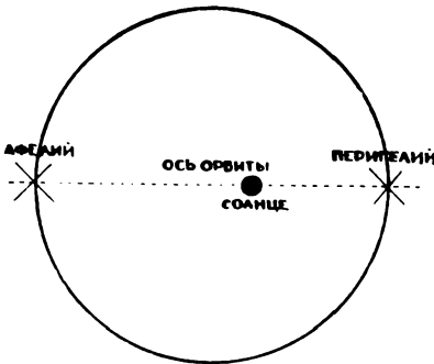
Орбита Меркурия вокруг Солнца. Черт. 4.
