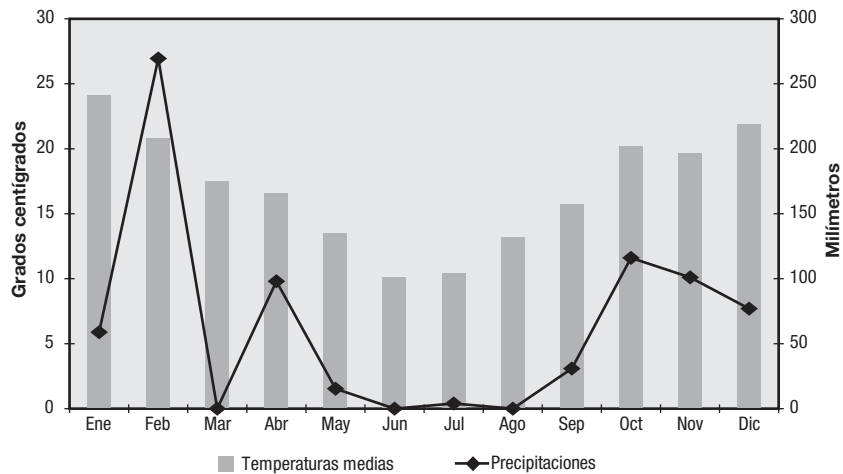
Gráfico 2. Precipitaciones y temperaturas medias mensuales por estación meteorológica de Córdoba. Año 2014
