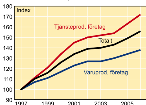
Arbetskraftskostnad, index 1997=100
