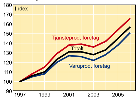
Förbrukningsvärde, index 1997=100
