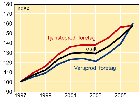
Produktionsvärde, index 1997=100
