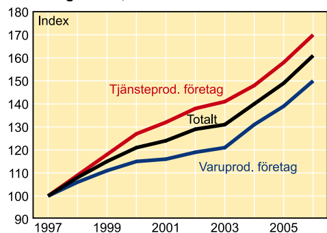
Förädlingsvärde, index 1997=100
