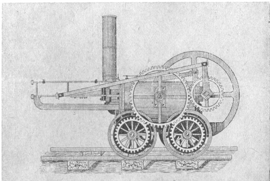
Паровоз Тревтика
