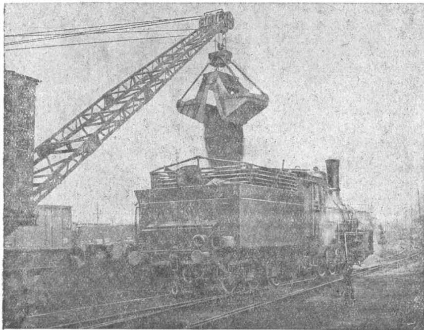
Снабжение паровоза углем грейферным краном
