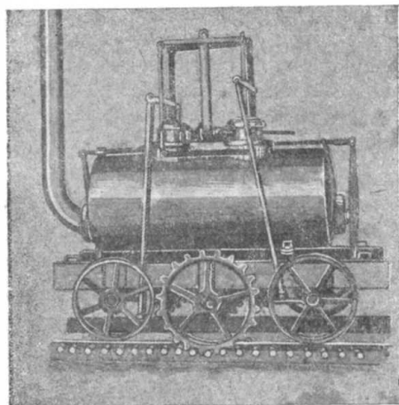
Паровоз Бленкинсопа
