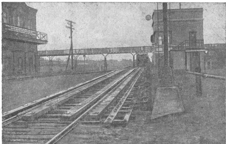
Механизованная горка
