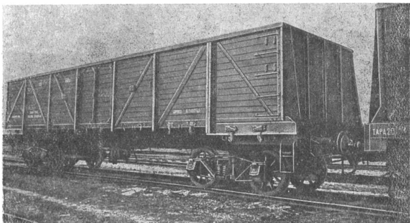
Саморазгружающийся полувагон-гондола
