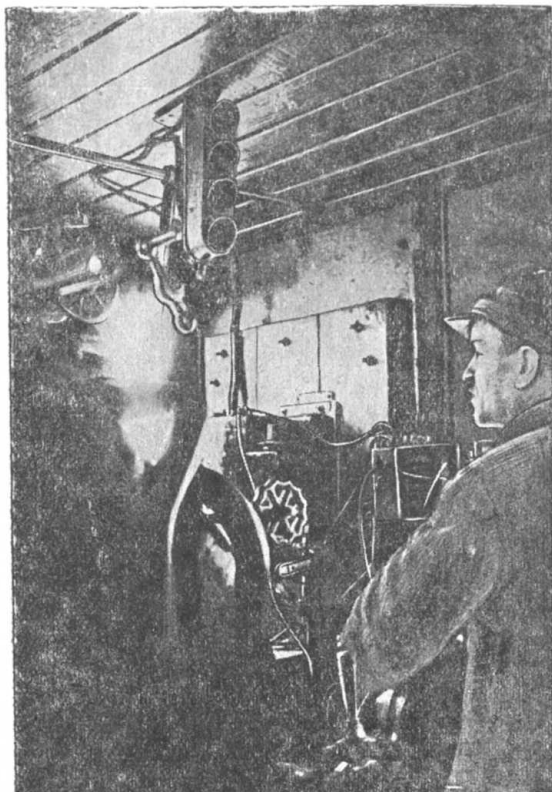
Кэб-сигнал
