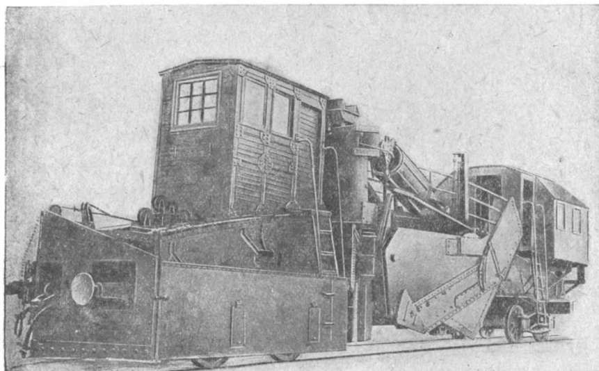
Путевой струг
