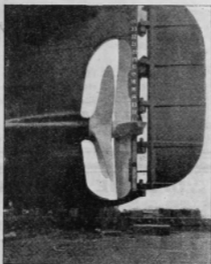
Изображение показывает Стар Контрапропеллер, установленный на 10.000-тонном пароходе
